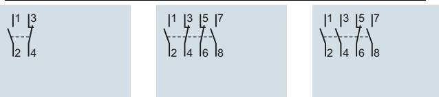
5TE8151 5TE8152 5TE8153
