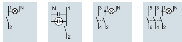
5TE8101 5TE8105 5TE8102 5TE8103 5TE8101-3
