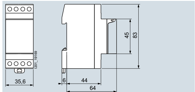
7LF451. 7LF452. 7LF453. 7LF454.
